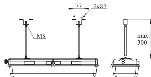
Montage met draadeind M6 Mounting with pendant M6
