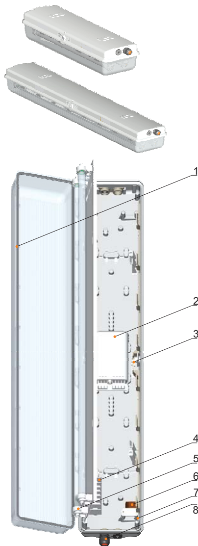
1 Afdichting t.b.v. beschermingsgraad IP 65 Gasket for protection degree IP65
